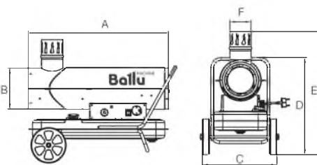
рис. 2 Размеры прибора
